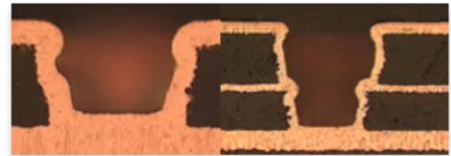
HDI Microvia
